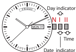
Cal. 8205/ 8285
